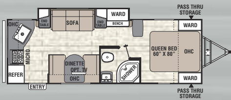
246 RKS / Longueur extérieure 28' 3"
