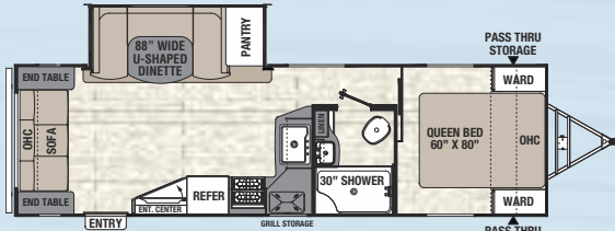
279 RLSLE / Longueur extérieure 31' 11"
