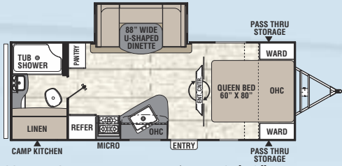
231 RBSLE / Longueur extérieure 26' 10"
