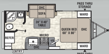
192 RBS / Longueur extérieure 22' 6"
