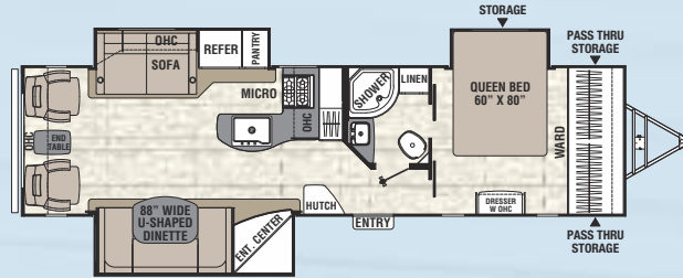
293 RLSLE / Longueur extérieure 35' 11"
