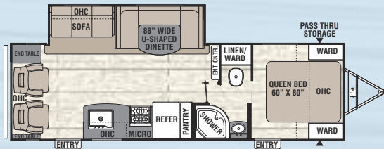
281 RLSLE / Longueur extérieure 31' 8"
