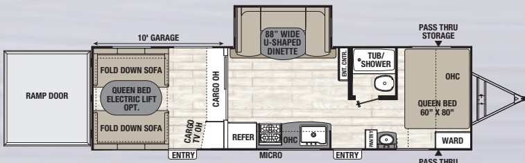
301 BLDS / Longueur extérieure 33' 7"
