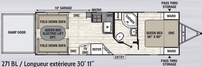
271 BL / Longueur extérieure 30' 11"
