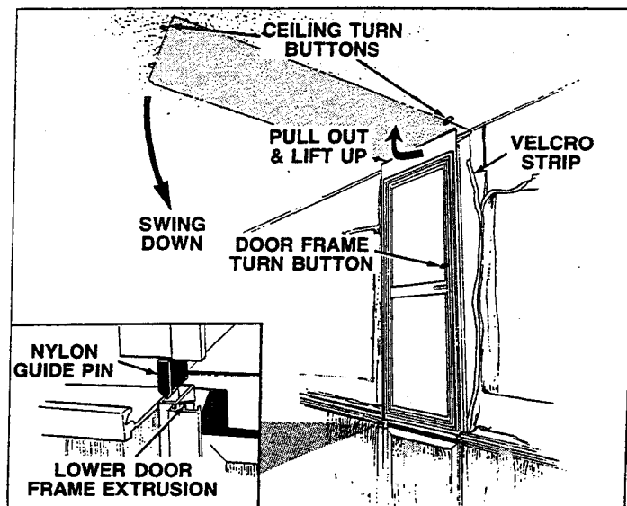
DOOR ASSEMBLY
